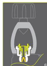
Figure C : Détendeur non connecté en étrier > détendeur obstrué
