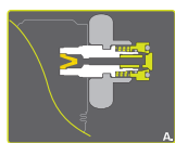
Figure A : Détendeur non connecté en Din > détendeur obstrué
