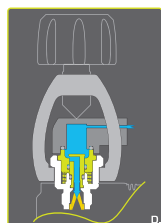
Figure D : Détendeur connecté en étrier > détendeur ouvert
